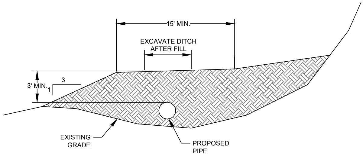
SECTION N.T.S.
