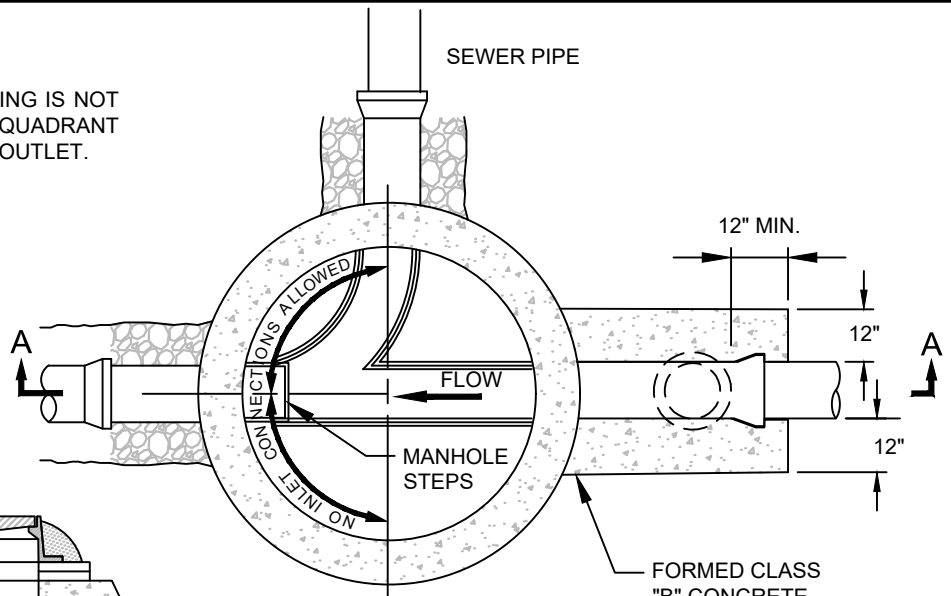
SECTIONAL PLAN N.T.S.
