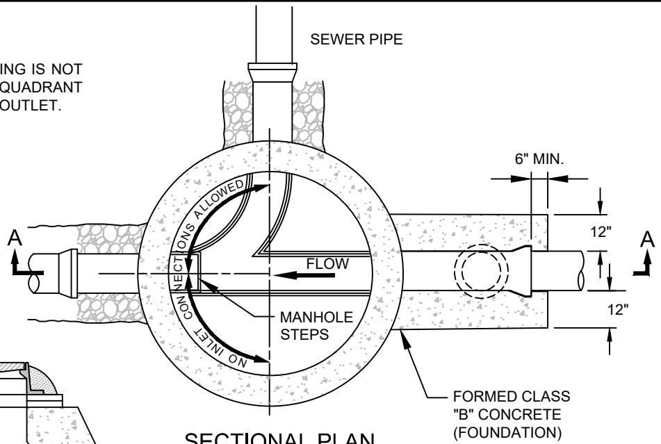
SECTIONAL PLAN N.T.S.
