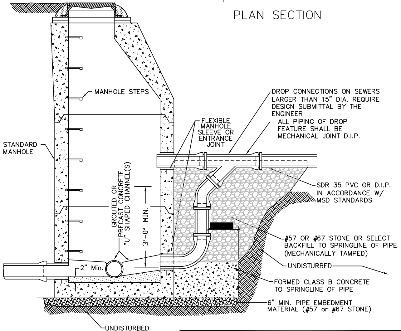
SECTION A-A
